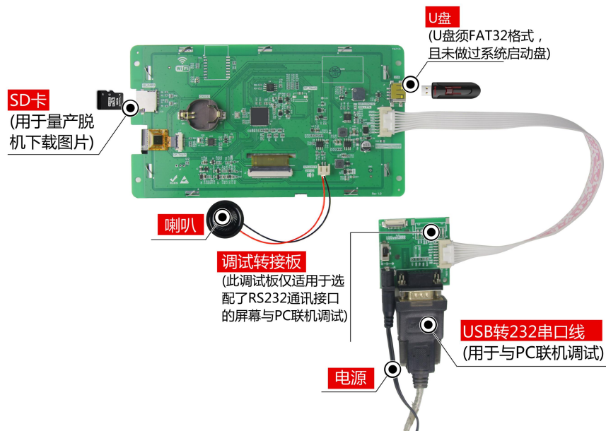
图 1-5 调试工具图
