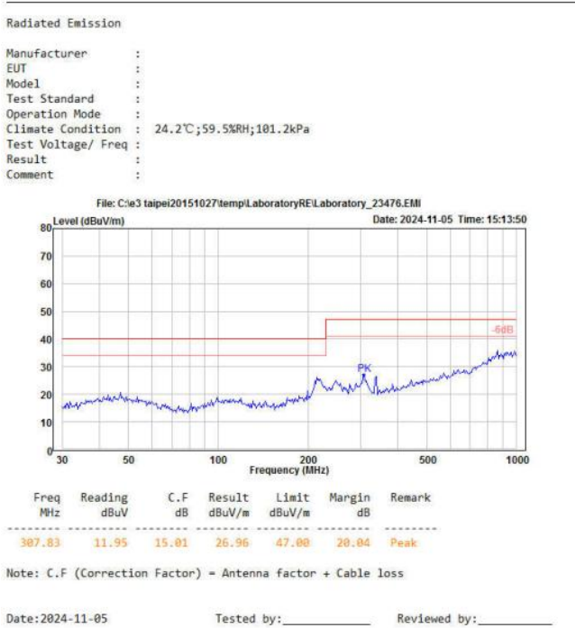
图 5-6 辐射测试水平方向
