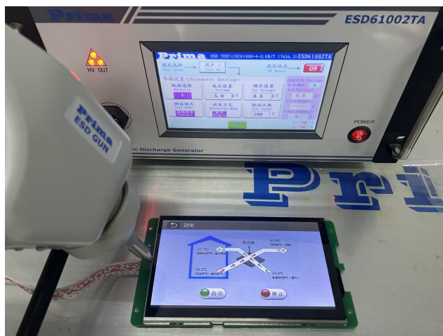
图 5-2 ESD 测试图
